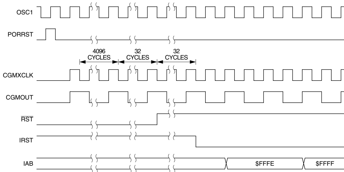
Figure 6-7. POR Recovery
